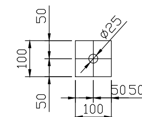
PEÇA 03 CHAPA # 3/8" QUANTIDADE = 08 PÇS.
