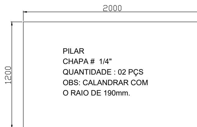
PILAR CHAPA # 1/4" QUANTIDADE : 02 PÇS OBS: CALANDRAR COM O RAIOS DE 190mm.
