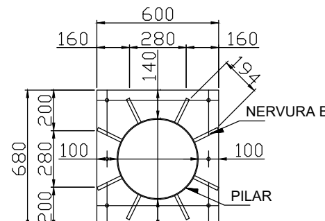
SEÇÃO BB
