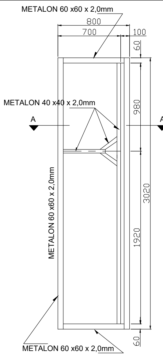
PLATAFORMA SECUNDÁRIA
