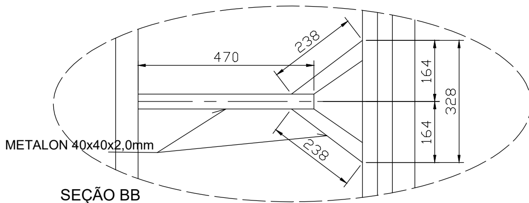
SEÇÃO BB
