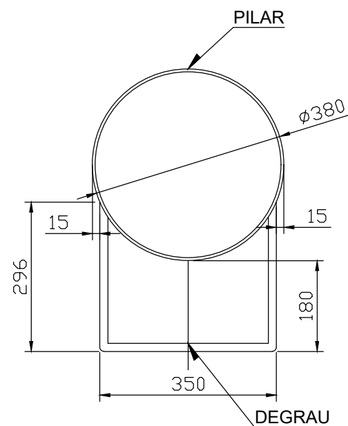
CORTE DO PILAR
