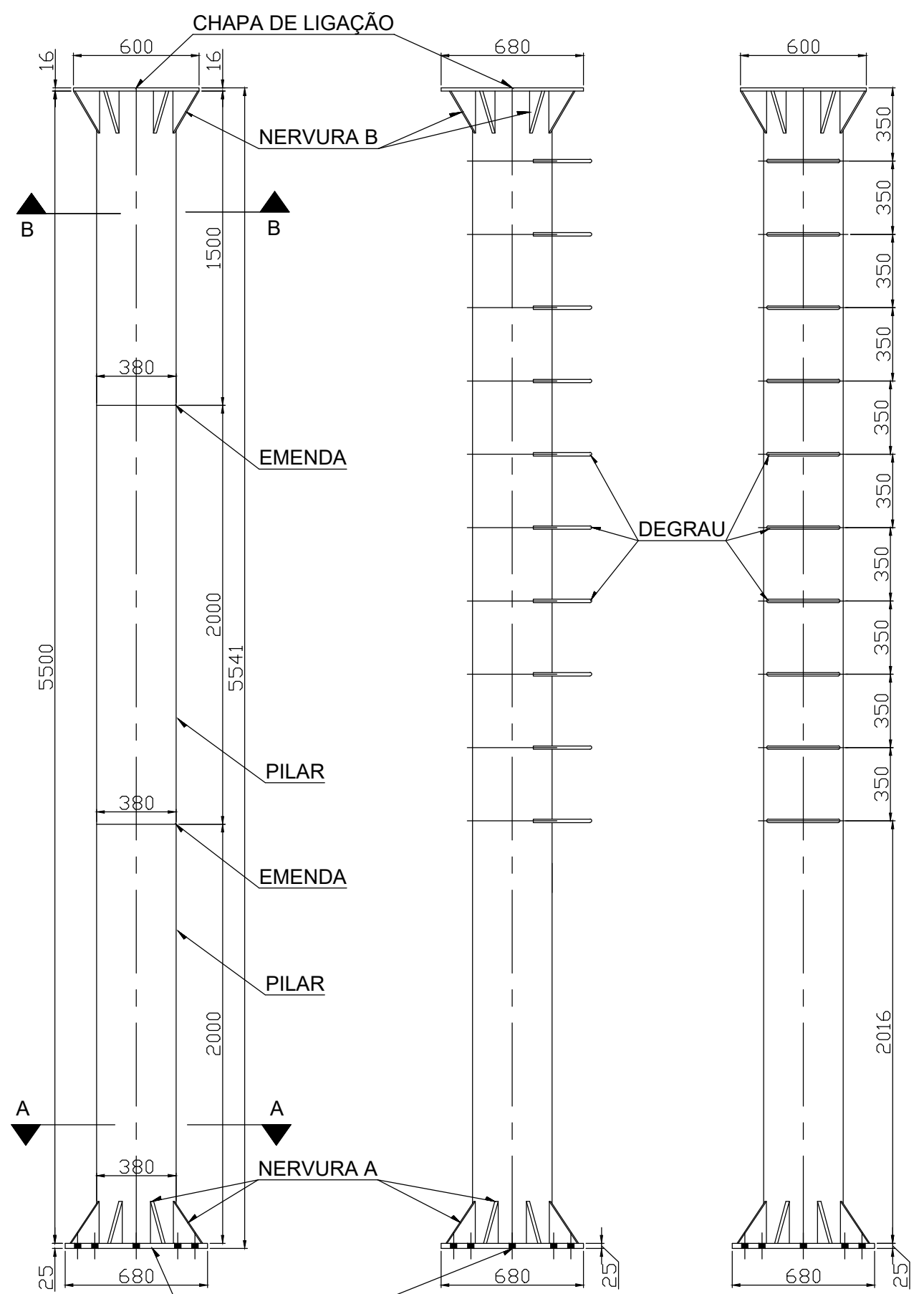
PILAR VISTA LATERAL
