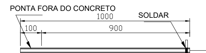
CHUMBADORES BARRA ROSQUEADA Ø 1" QUANTIDADE = 08 PÇS.
