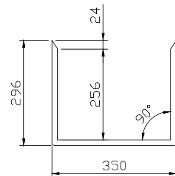
DEGRAU FERRO REDONDO Ø 5/8" QUANTIDADE: 10 PÇS
