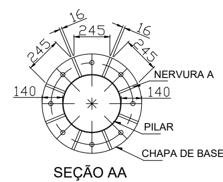
SEÇÃO AA
