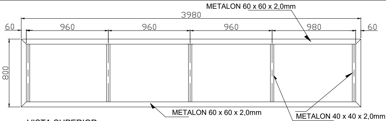
VISTA SUPERIOR
