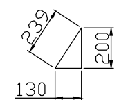
NERVURA B CHAPA # 5/8" QUANTIDADE : 08 PÇS
