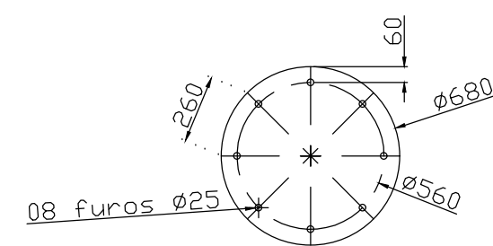
CHAPA GABARITO CHAPA # 1/8" QUANTIDADE: 01 PÇ
