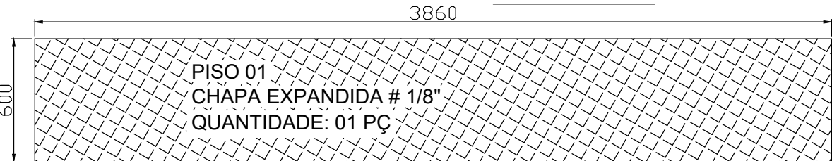
PLATAFORMA SECUNDÁRIA
