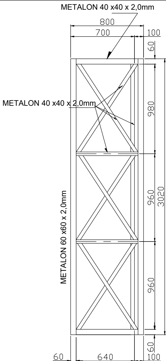
VISTA LATERAL
